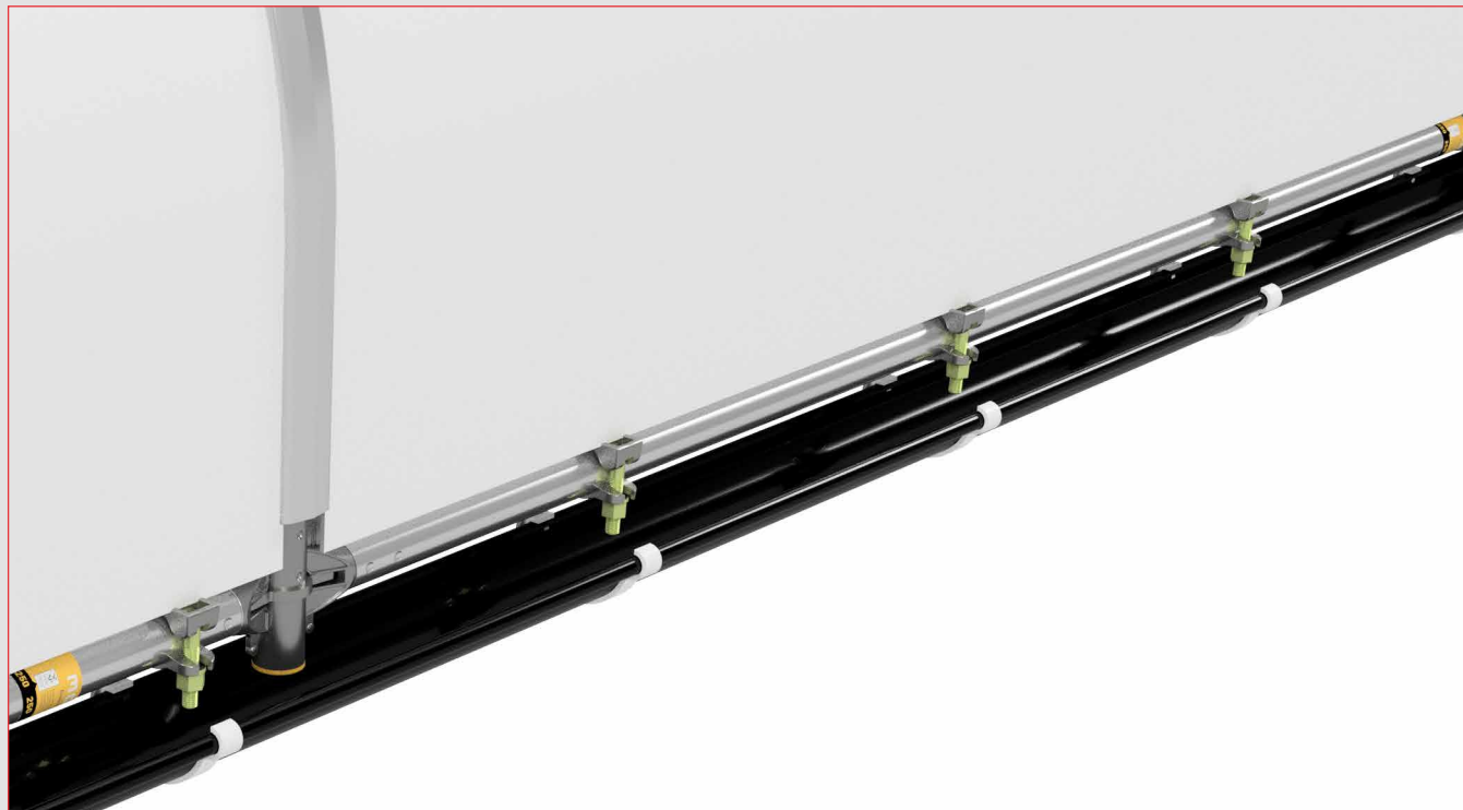
屋根排水システムで汎用125 mm雨樋用雨樋 Bracketを使用して屋根から雨水を集めます。
